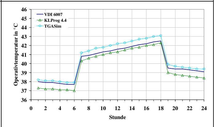
Bild 4: Testbeispiel 1, Operativtemperatur, 10. Tag
