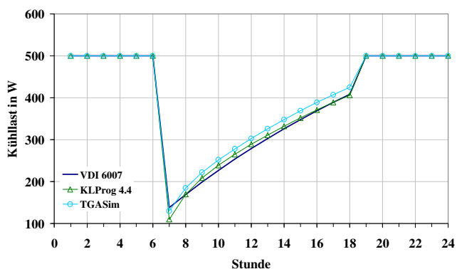
Bild 35: Testbeispiel 7, Kühllast, 10. Tag
