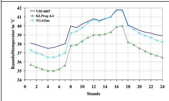
Bild 44: Testbeispiel 9, Raumlufthemperatur, 10. Tag
