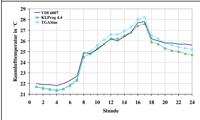
Bild 42: Testbeispiel 9, Raumlufthemperatur, 1. Tag
