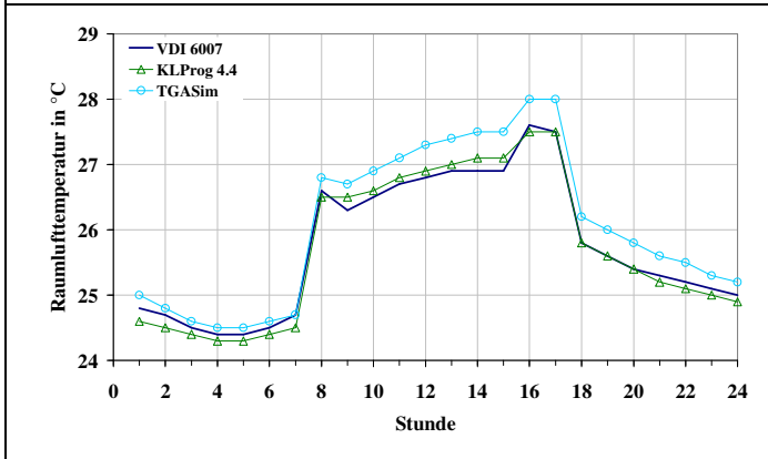
Bild 50: Testbeispiel 10, Raumlufttemperatur, 10. Tag
