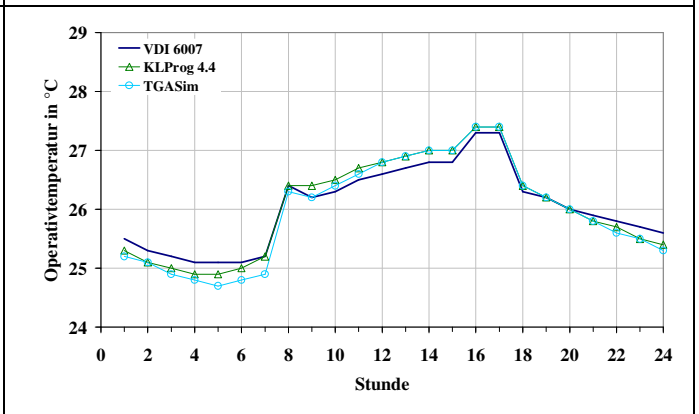
Bild 53: Testbeispiel 10, Operativtemperatur, 60. Tag
