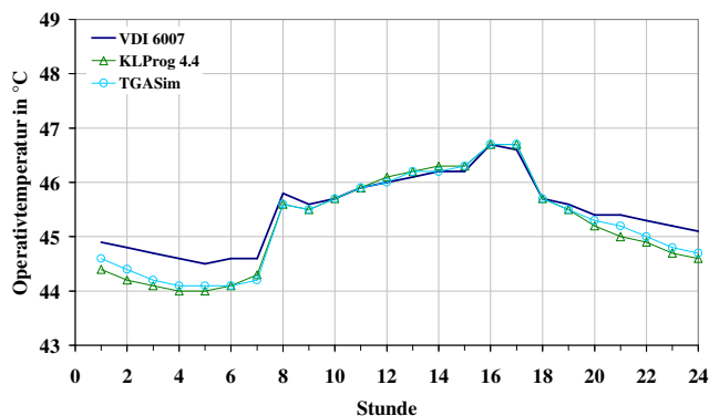
Bild 30: Testbeispiel 5, Operativtemperatur, 60. Tag
