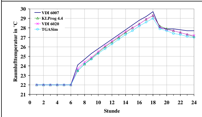
Bild 19: Testbeispiel 4, Raumlufttemperatur, 1. Tag
