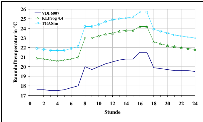
Bild 48: Testbeispiel 10, Raumlufttemperatur, 1. Tag
