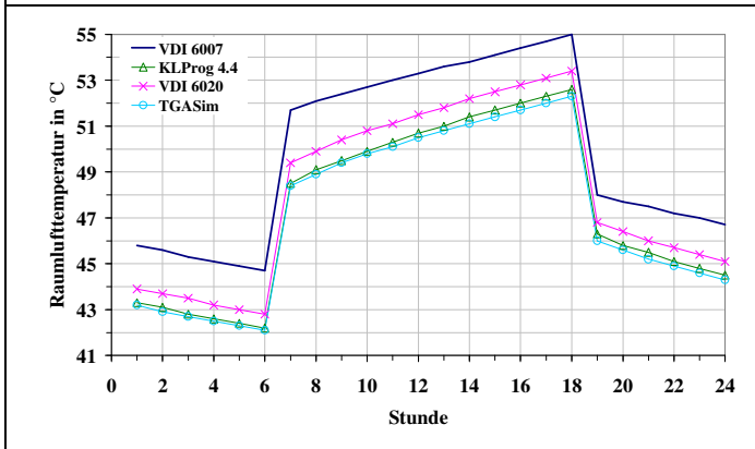
Bild 15: Testbeispiel 3, Raumlufthemperatur, 10. Tag
