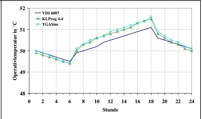
Bild 12: Testbeispiel 2, Operativtemperatur, 60. Tag
