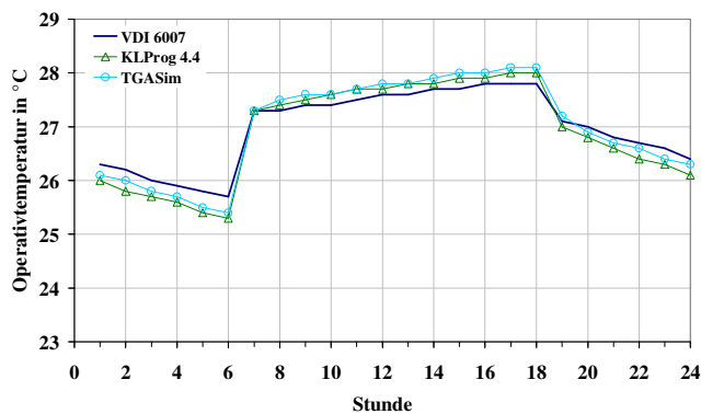
Bild 34: Testbeispiel 7, Operativtemperatur, 10. Tag
