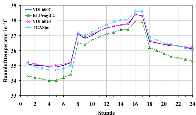
Bild 27: Testbeispiel 5, Raumlufthemperatur, 10. Tag
