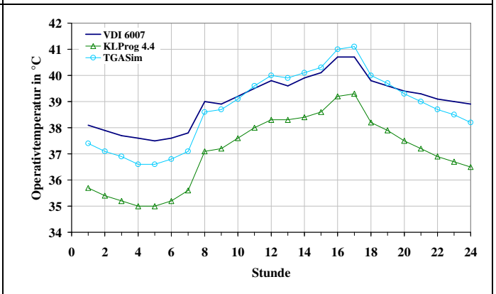
Bild 45: Testbeispiel 9, Operativtemperatur, 10. Tag
