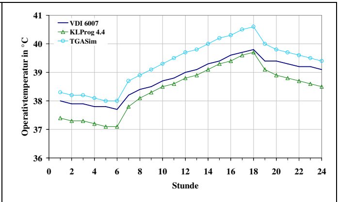
Bild 10: Testbeispiel 2, Operativtemperatur, 10. Tag
