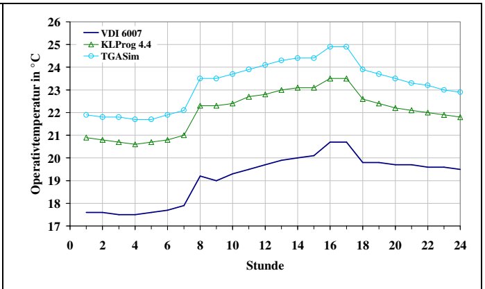
Bild 49: Testbeispiel 10, Operativtemperatur, 1. Tag
