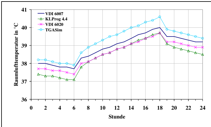
Bild 9: Testbeispiel 2, Raumlufthemperatur, 10. Tag
